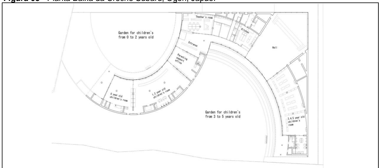
Figura 08 - Planta Baixa da Creche Subaru, Ogori, Japão.
